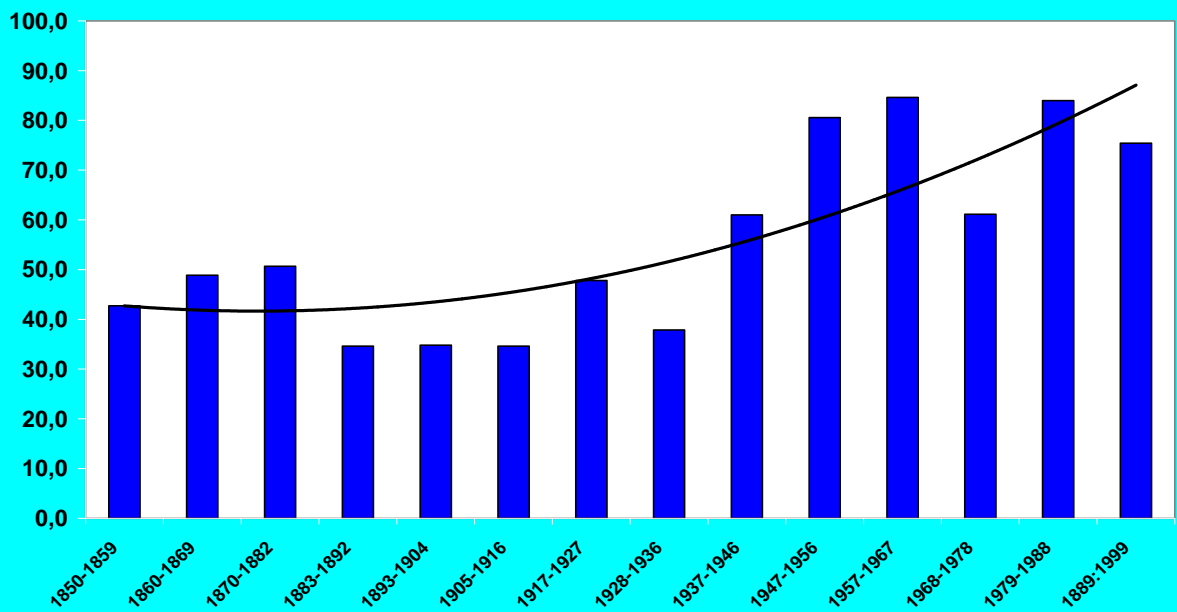
Abb. 2 Mittlere Sonnenfleckenanzahl je Sonnenfleckenzyklus 1850 - 1999
