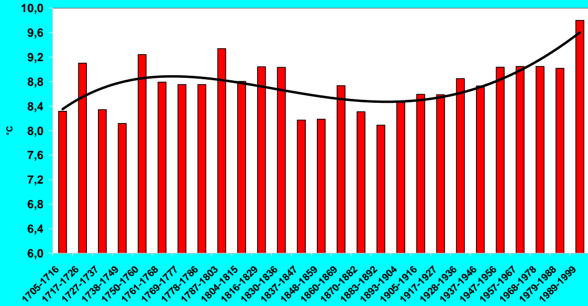
Abb. 3 Mitteltemperaturen je Sonnenfleckenzyklus von Mitteleuropa 1705 - 1999
