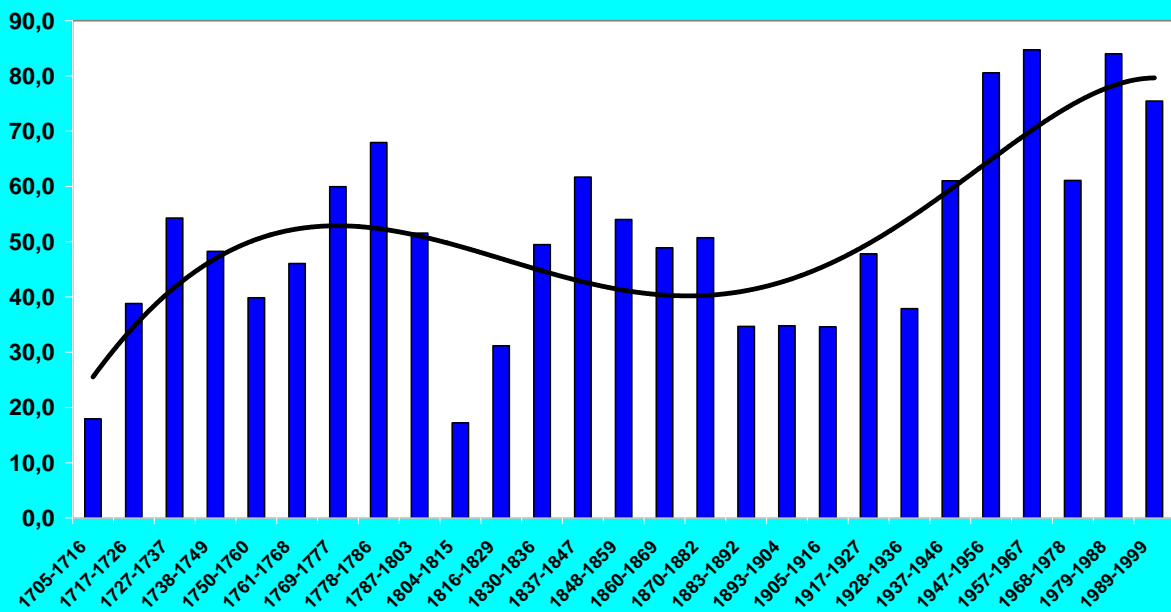
Abb. 4 Mittlere Sonnenfleckenanzahl je Sonnenfleckenzyklus 1705 - 1999
