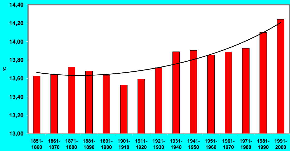
Abb. 1 10-jährige globale Temperaturentwicklung 1851 - 2000
